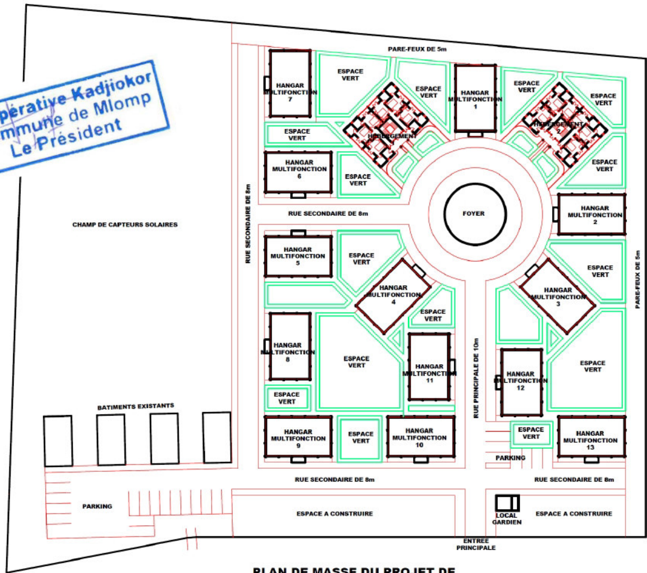
PLAN DE MASSE DU PROJET DE CONSTRUCTION DU CENTRE DE MLOMP
